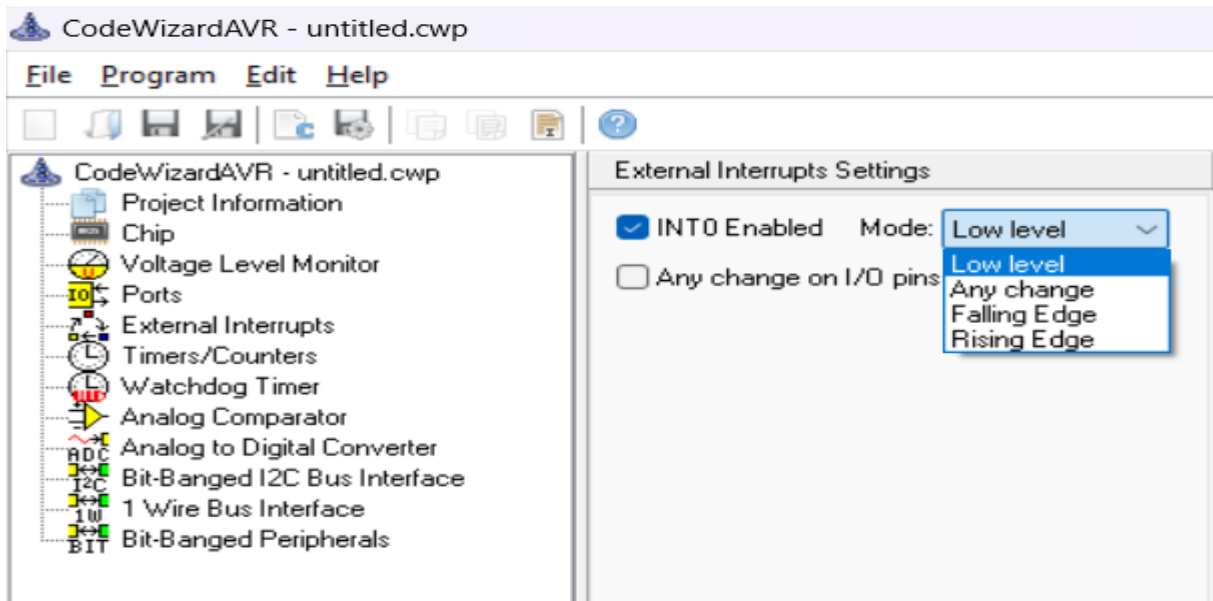
شکل ۳- سربرگ وقفه خارجی
