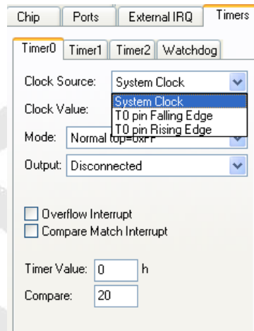
شکل ۶- انتخاب منبع پالس برای شمارنده
