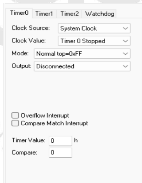
شکل ۴- سربرگ تایمر
