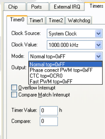
شکل ۵- مدهای کاری مربوط به Timer0
